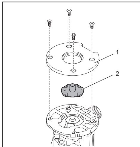
► 1. Plaque de base 2. Guide de gabarit
