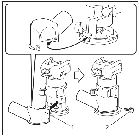
► 1. Dust nozzle 2. Thumb screw
