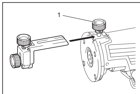
► 1. Clamp screw
