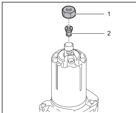
► 1. Collet nut 2. Collet cone
