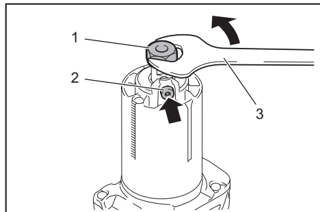
► 1. Écrou de mandrin 2. Verrou d'arbre 3. Clé
