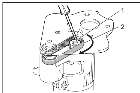
► 1. Poulie 2. Courroie
