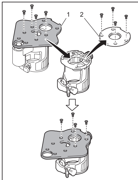
► 1. Plaque de base désalignée 2. Plaque de base d'affleureuse
