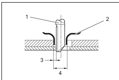
► 1. Embout pour affleureuse 2. Guide de gabarit 3. Distance (X) 4. Diamètre extérieur du guide de gabarit
