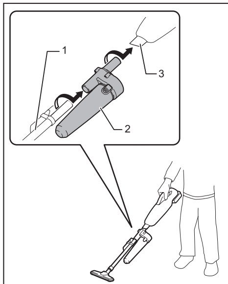
► 1. Tuyau rectiligne 2. Collecteur cyclone 3. Entrée d'aspiration
