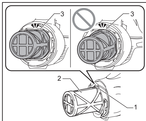
► 1. Rainure du boîtier d'aspirateur 2. Préfiltre 3. Rebord de fixation
