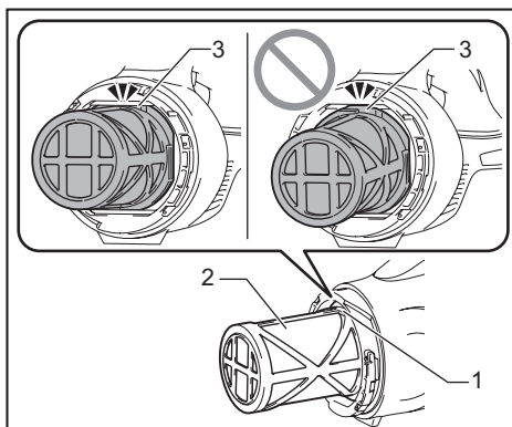
► 1. Ranura de la carcasa de la aspiradora 2. Prefiltro 3. Reborde de fijación
