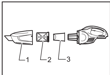
► 1. Bac à poussière 2. Préfiltre 3. Filtre
