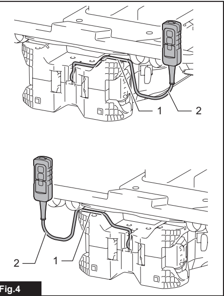
► 1. Rainure 2. Cordon
