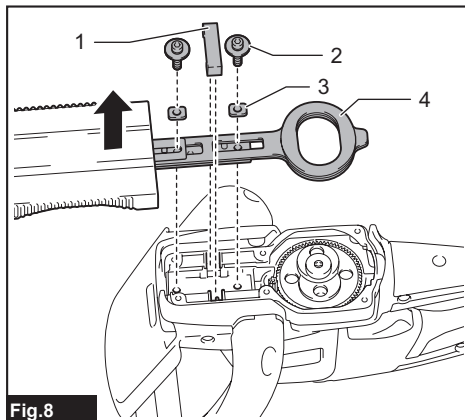
► 1. Coussinet de feutre 2. Boulon 3. Manchon 4. Lames de cisaillement
