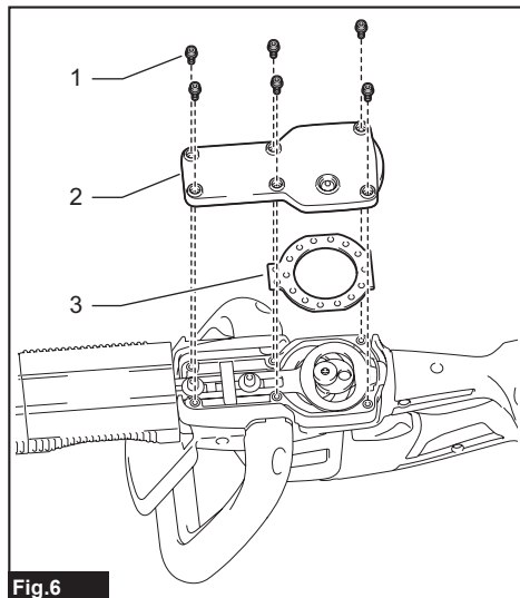
► 1. Boulon 2. Couvercle 3. Plaque
