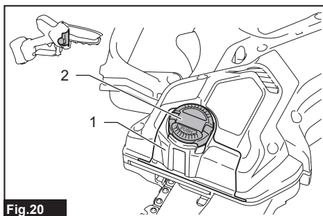
► 1. Fenêtre de vérification du niveau d'huile 2. Bouchon du réservoir d'huile
