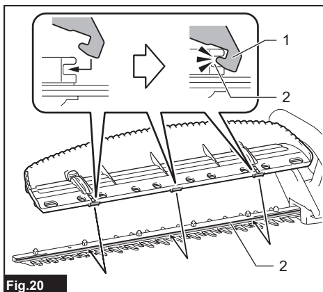
► 1. Griffes 2. Rainure
