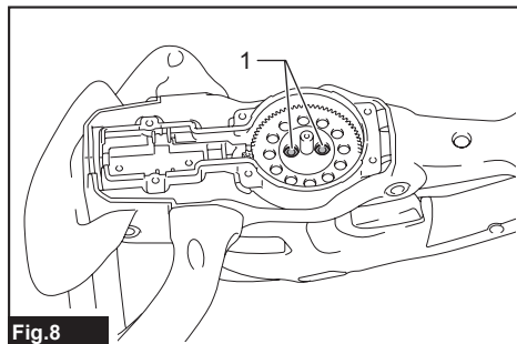
► 1. Resin sleeve
