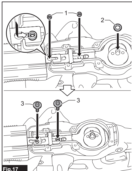
► 1. Manchon métallique 2. Rondelle plate 3. Boulon
