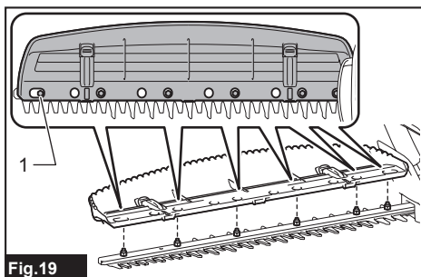
► 1. Vis
