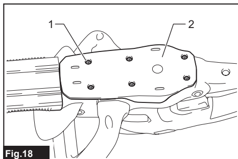
► 1. Vis 2. Couvercle
