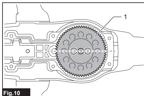
► 1. Gear
