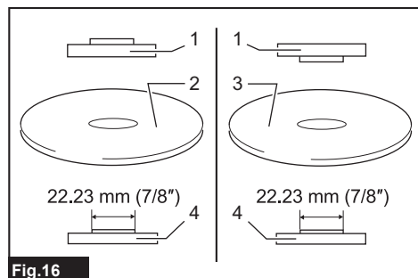
Fig.16 ► 1. Contre-écrou 2. Meule tronçonneuse abrasive (plus mince que 4 mm (5/32")) 3. Meule tronçonneuse abrasive (4 mm (5/32)) ou plus épaisse 4. Flasque intérieur
