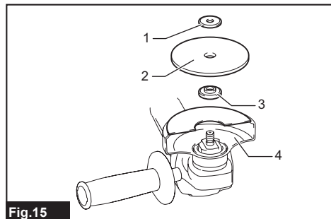
Fig.15 ► 1. Contre-écrou 2. Meule tronçonneuse abrasive / meule diamant 3. Flasque intérieur 4. Protecteur de meule pour meule tronçonneuse abrasive / meule diamant
