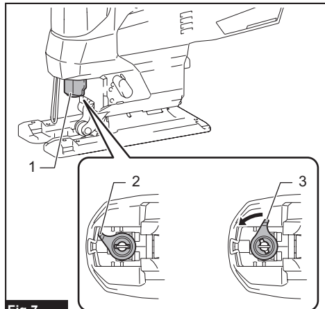
Fig. 7 ▶ 1. Porte-lame de scie sauteuse 2. Levier de serrage de lame (position libérée) 3. Levier de serrage de lame (position fixée)
